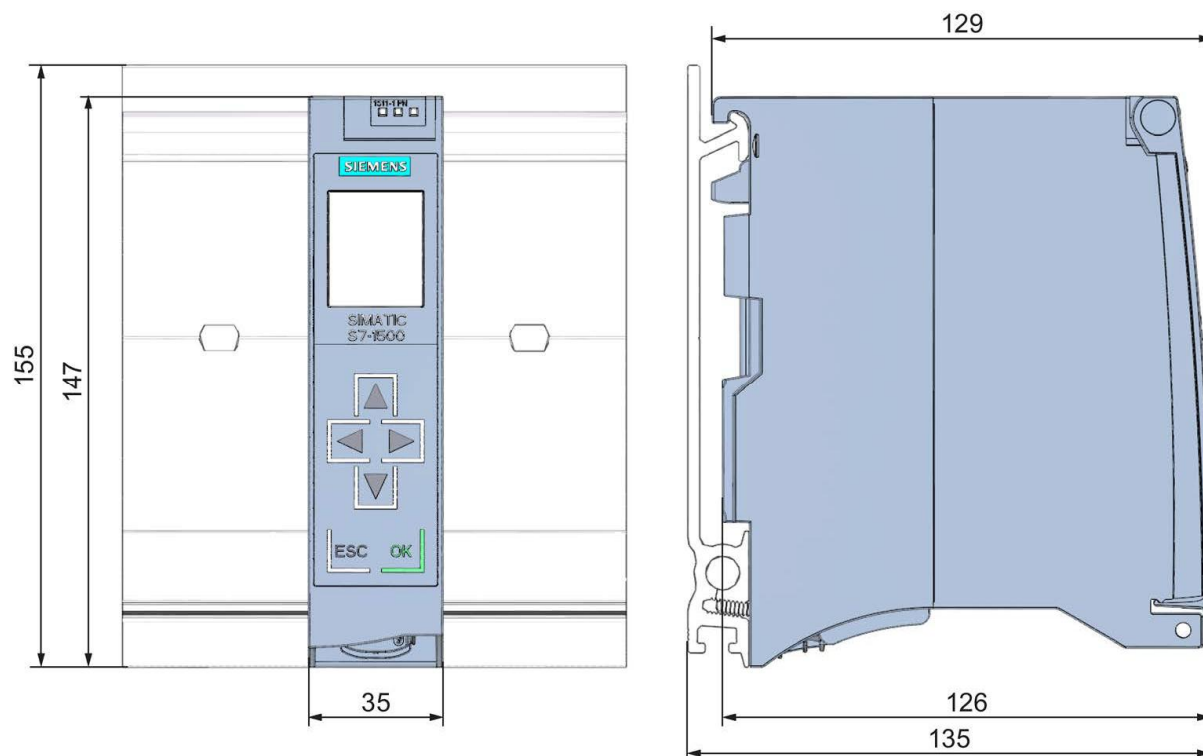
Рисунок А-1 Габаритный чертеж CPU 1511-1 PN, вид спереди и вид сбоку
