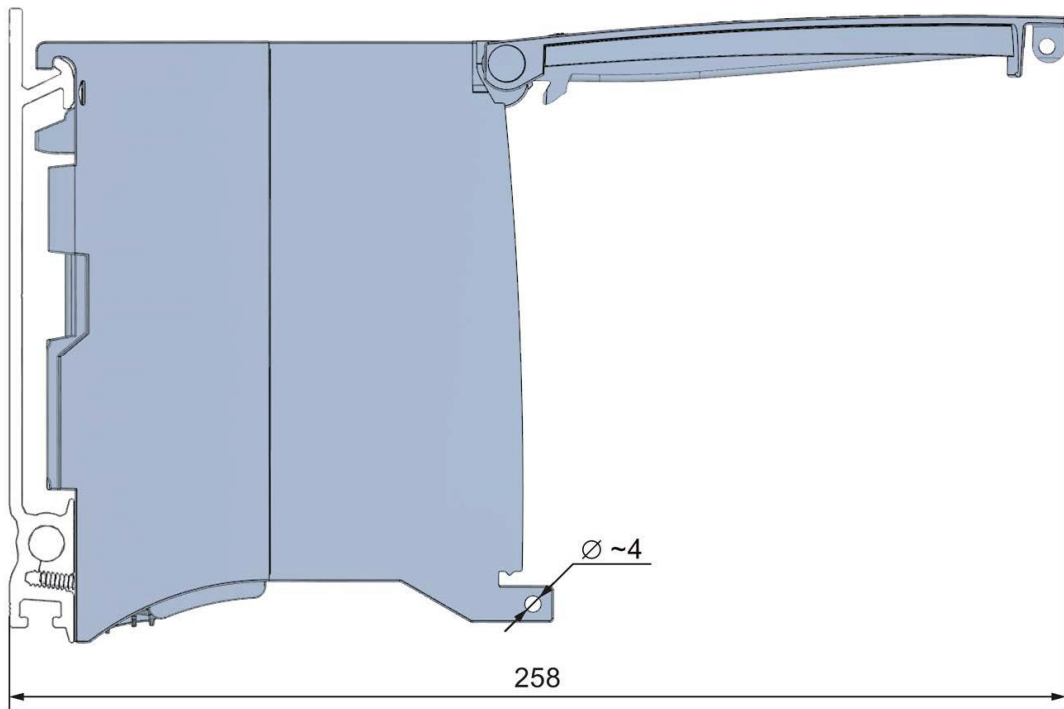
Рисунок А-2 Габаритный чертеж CPU 1511-1 PN, (вид сбоку, открытой передней крышкой)
